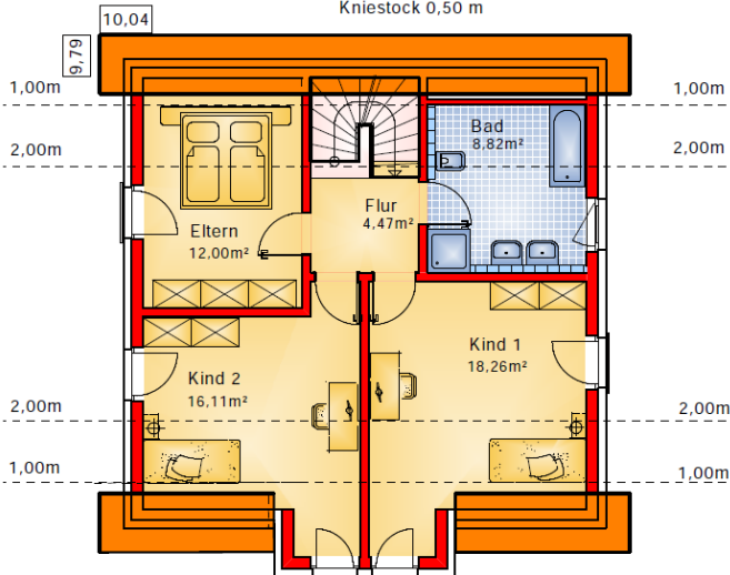
Dachneigung 38° Kniestock 0,50 m
